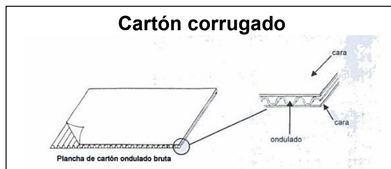
Ilustración 3 - Sección esquemática del cartón ondulado 10
